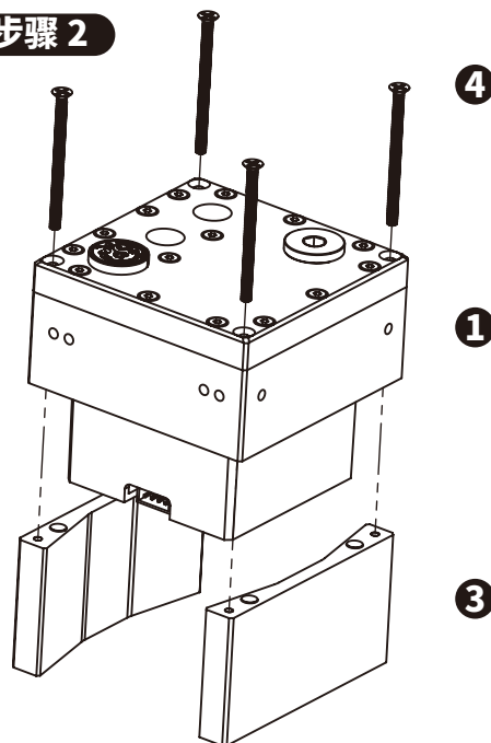
安装垫高支架
