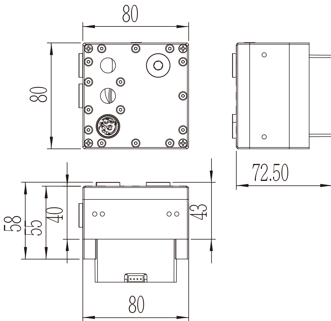
尺寸參考
