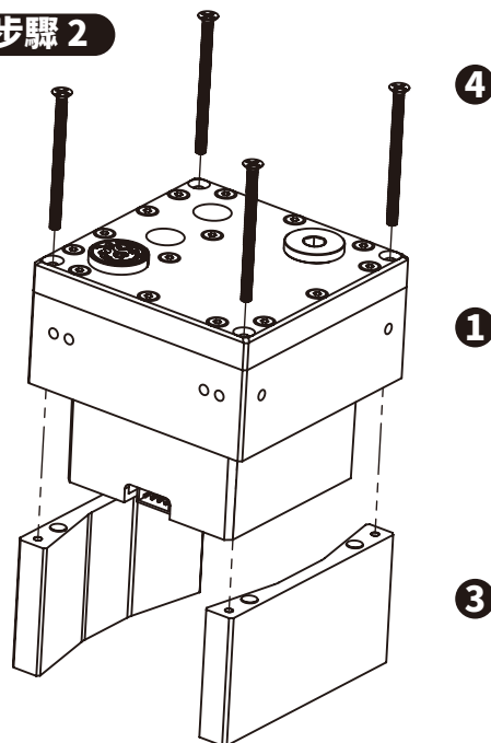
安裝墊高支架
