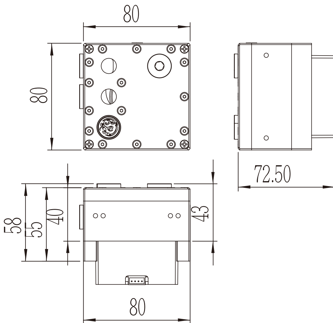
尺寸参考
