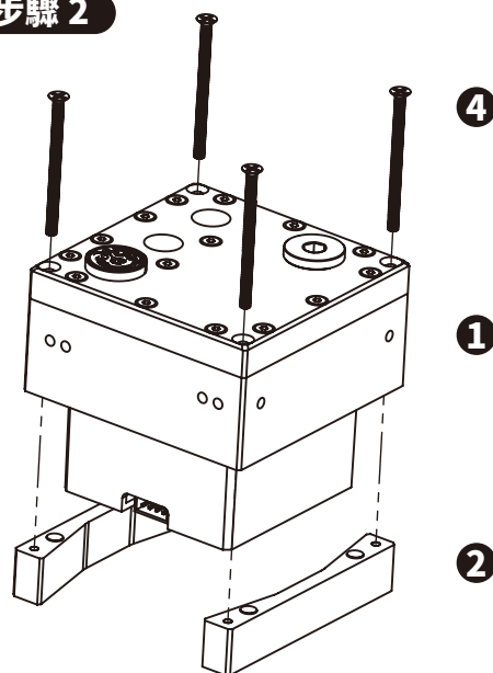
安裝固定支架
